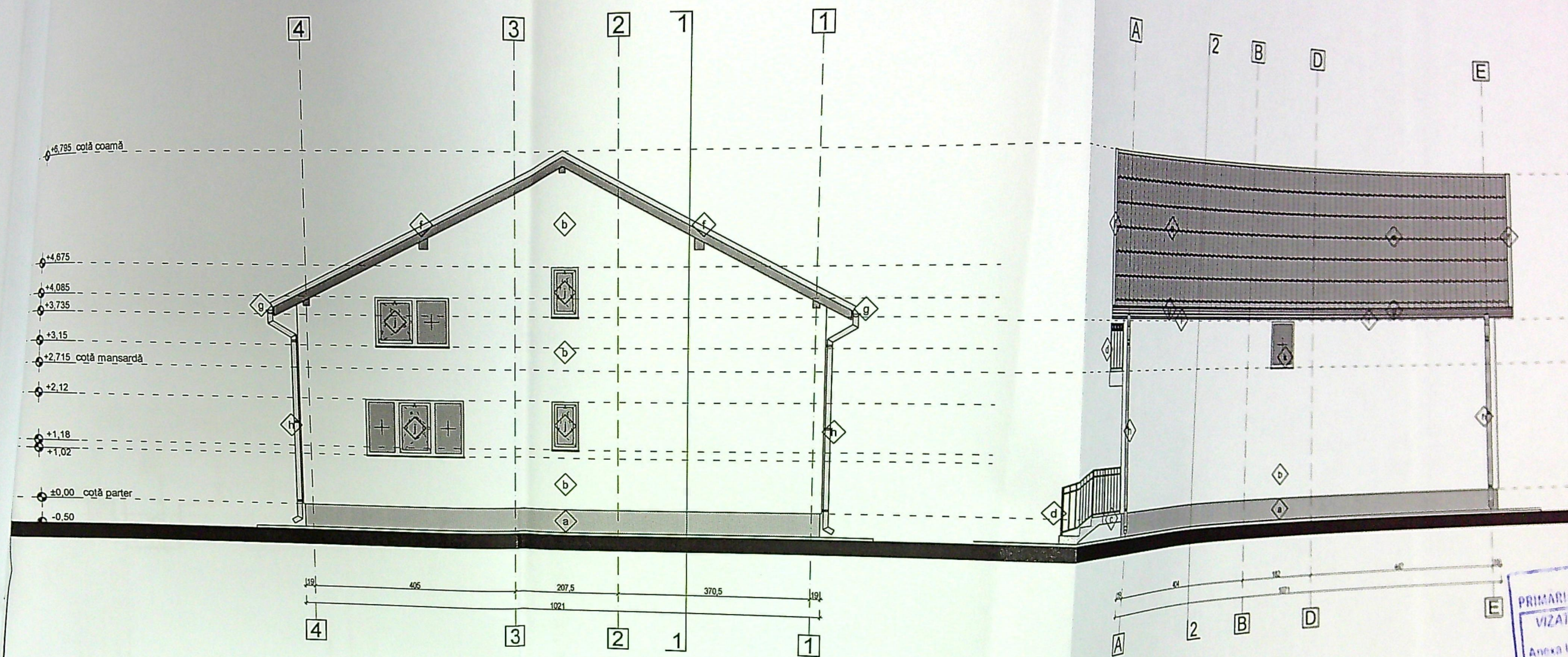
FAȚADĂ SUD-VEST sc. 1:100
