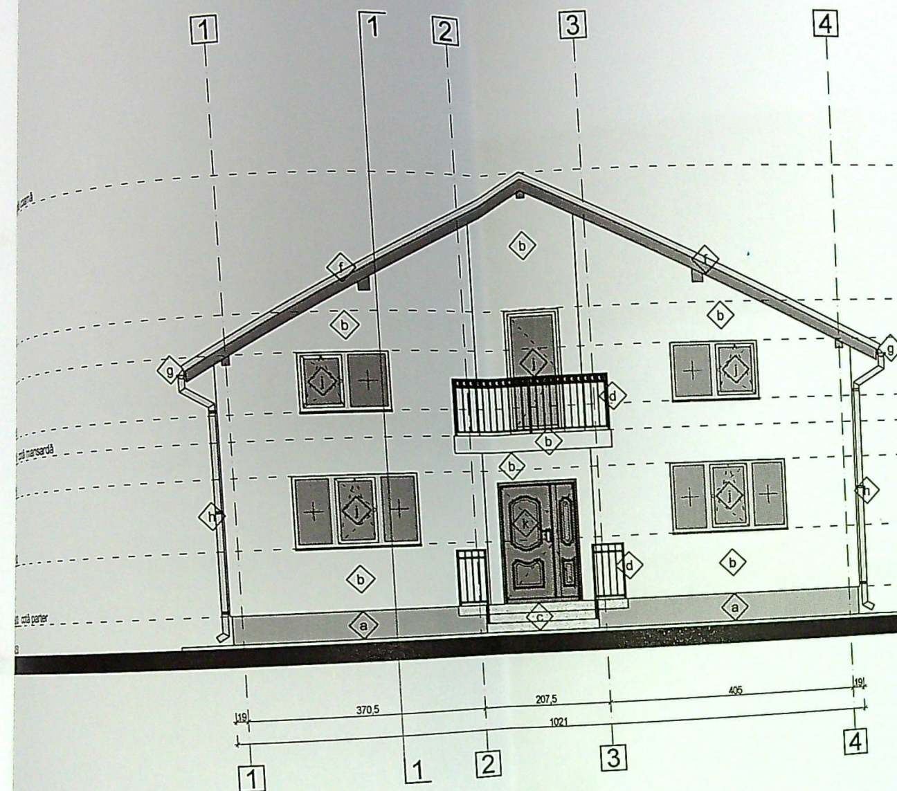
FAȚADĂ NORD-EST sc. 1:100
