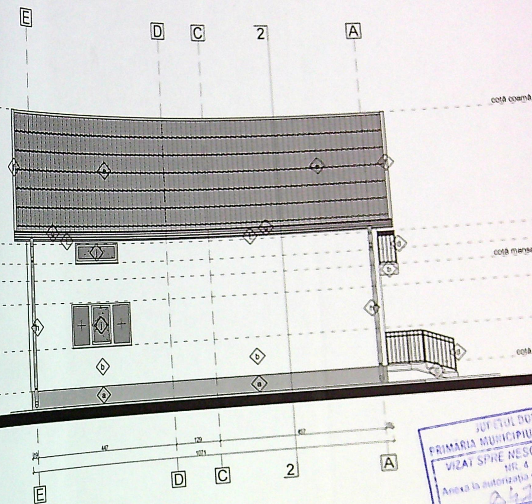
FAȚADĂ SUD-EST sc. 1:100
